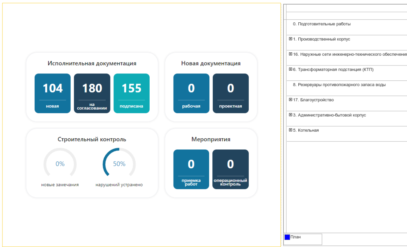
Рисунок 176 – Монитор проекта
